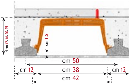
TEGOPLAST in sezione montato su travetti c.a.p.
